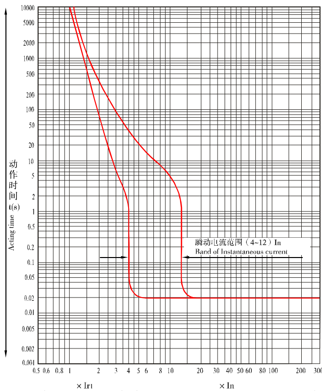
CM2-400L、M、H时间/电流特性曲线（配电）
