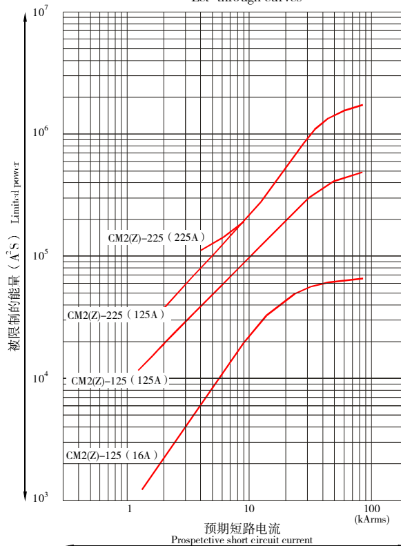
CM2(Z)-125、CM2(Z)-225 允通曲线
