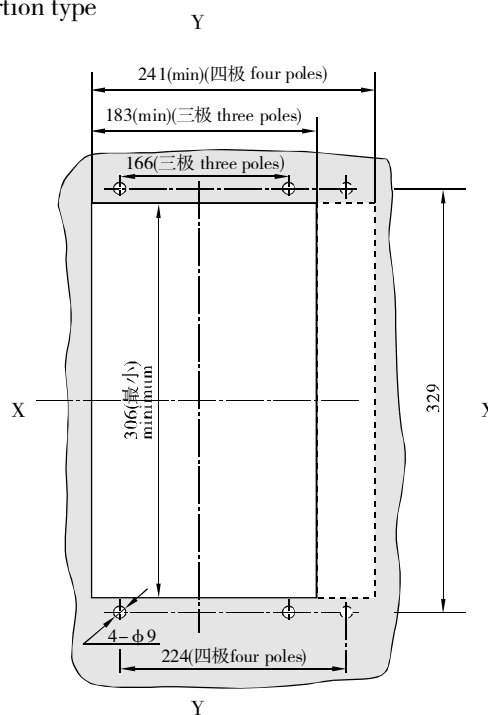
安装方式二开孔尺寸
