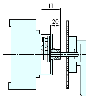
CM2 CM2Z -125、225、400、630
