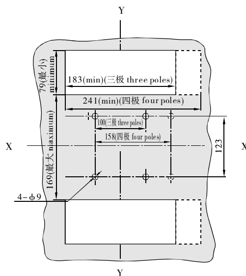
安装方式一开孔尺寸
