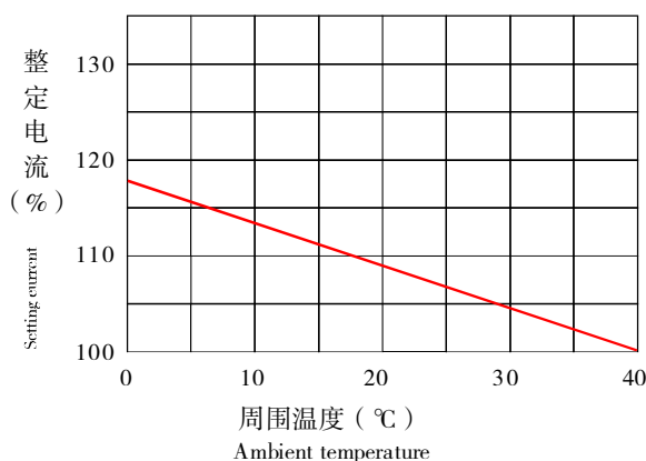
电流-温度特性
