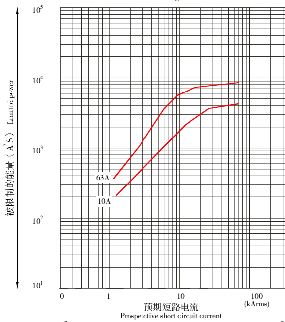
CM2-63 允通曲线
