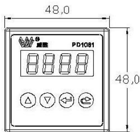
正视图
