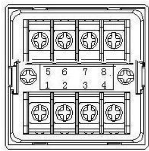
后视图
