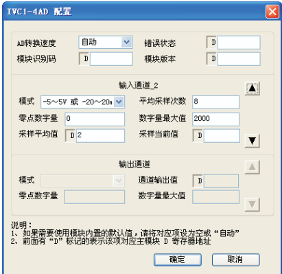
图 4-3 二号通道设置界面
