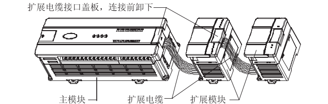
图 1-3 与主模块和其他扩展模块的连接示意图
