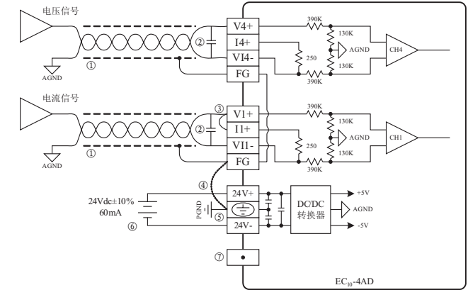
图 1-4 用户端子布线示意图
