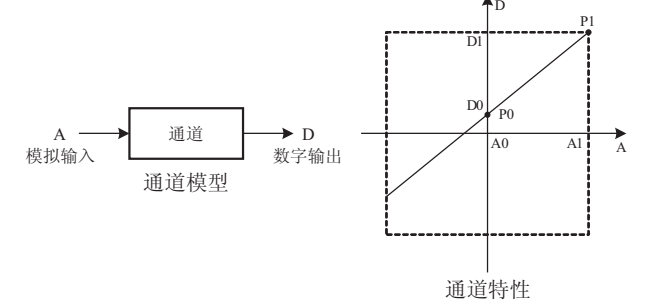
图 3-1 IVC1-4AD 的通道特性示意图
