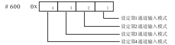
图 2-1 模式设定单元与通道对应关系
