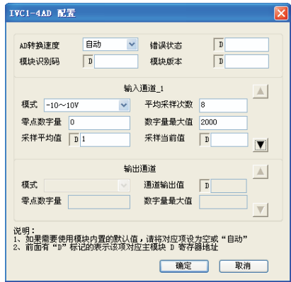
4-2 一号通道设置界面
